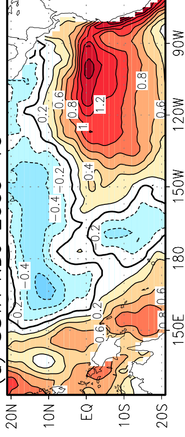
(d) SSTA NDJ 2009-10
