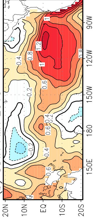
(b) SSTA FMA 2010
